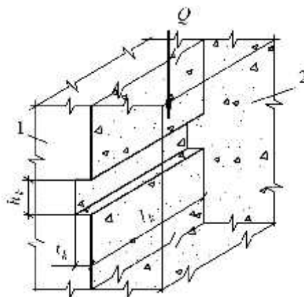
1 – сборный элемент; 2 – монолитный бетон
